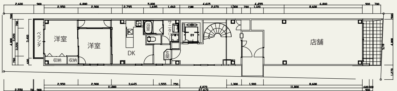
▲ 1階図面
