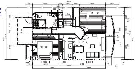
202,302,402号室
