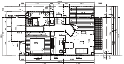
102号室
