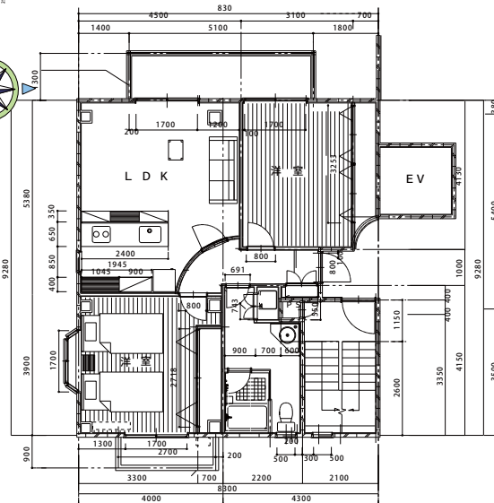
203号室
